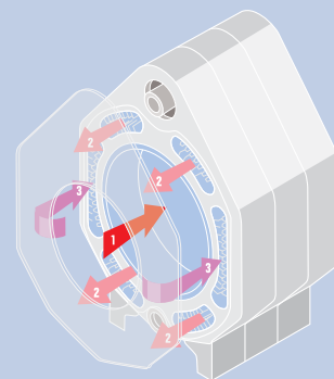
1-й проход продуктов сгорания 2-й проход продуктов сгорания 3-й проход продуктов сгорания
